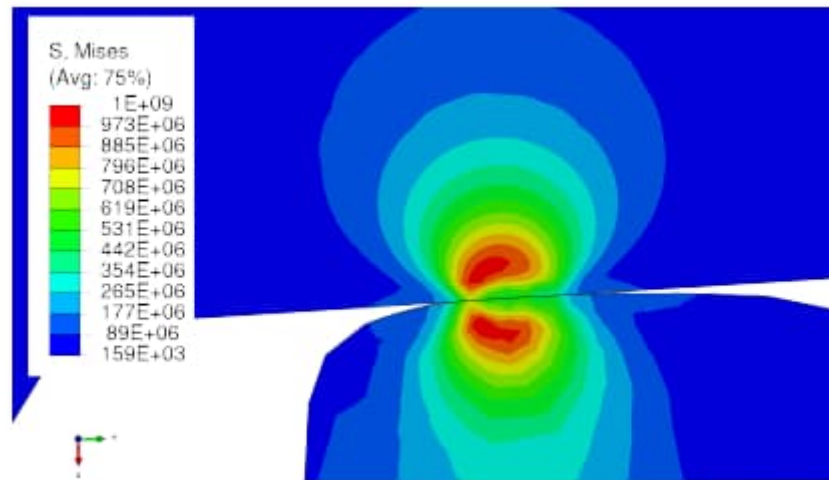
Figura 3 – Distribuição de tensão de Von Mises (Pa) na região de contato do modelo rodatrilho após o tratamento elástico (Fonte: Lima, 2018)
